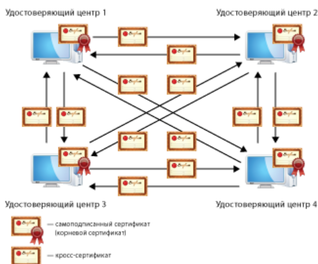
Рисунок 148. Распределенная модель доверительных отношений
