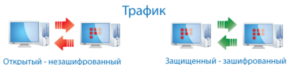
Рисунок 47. Виды IP-трафика
