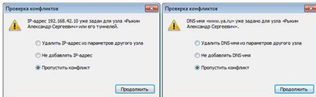
Рисунок 133. Действия при обнаружении пересечения IP-адресов или DNS-имен
