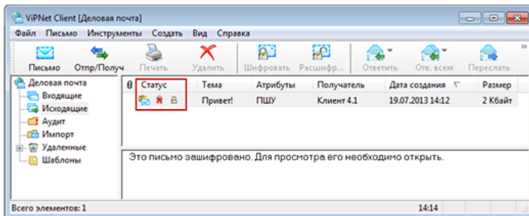
Рисунок 182. Новая колонка для отображения статуса письма
