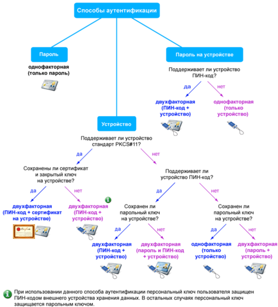
Рисунок 23. Схема соответствия между факторами и способами аутентификации
