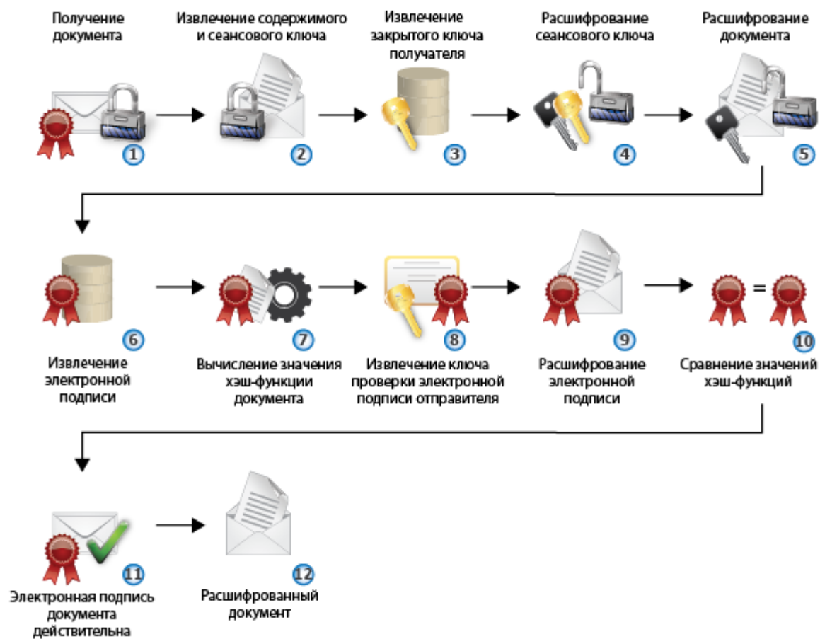
Рисунок 154. Процесс расшифрования и проверки электронного документа
